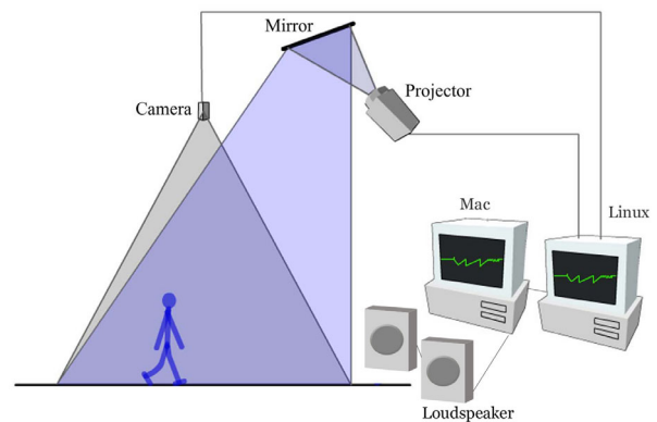
図 1: i-trace を用いた合奏システムの構成
