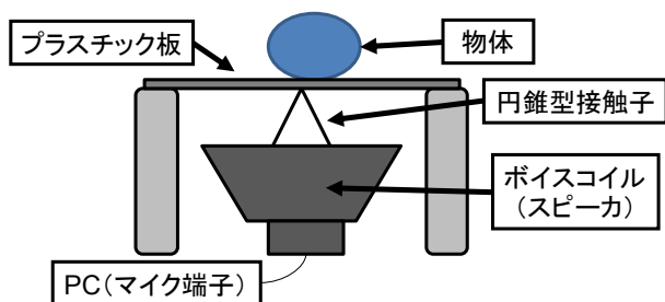
図2 振動計測台
