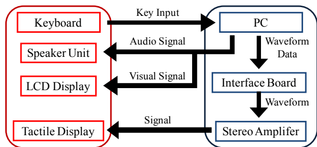
図3 再生システム
