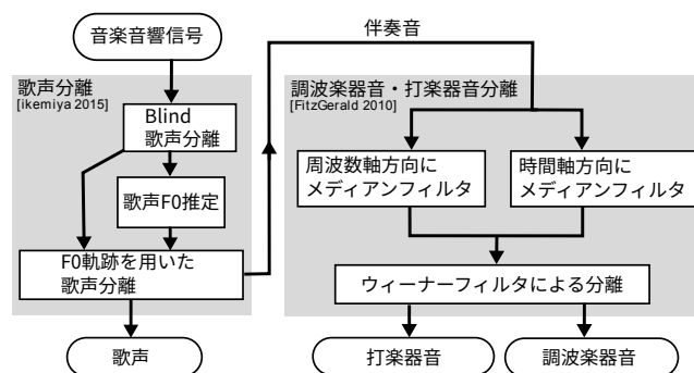
図 4 歌声・調波楽器音・打楽器音分離。
