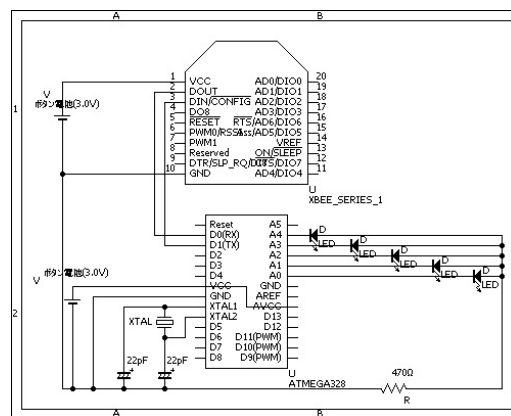
図5 光センサデバイス回路図
