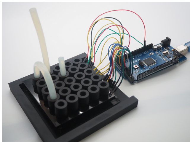
図4 デバイスの全体図
