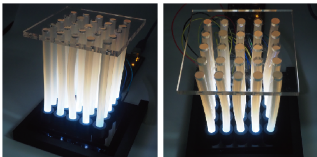
図 7 マトリクス型ディスプレイの表現例 1. 斜めから見た図 (左). 上から見た図 (右).
