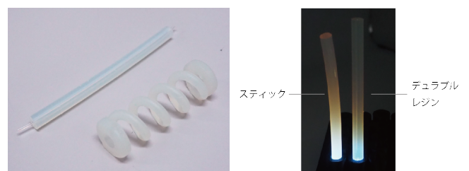
図 14 デュラブルレジンで造形した例 (左)。スティックとデュラブルレジンの点灯の比較 (右)。
