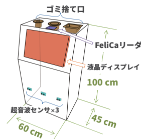
図 2 PoiPet の構造 Fig. 2 Structure of PoiPet
