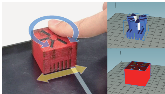
図 5 ダイヤルインタフェース外観。円形に配置された複数の導電部がオブジェクト内部を通して、底面の縞模様へ接続される。
