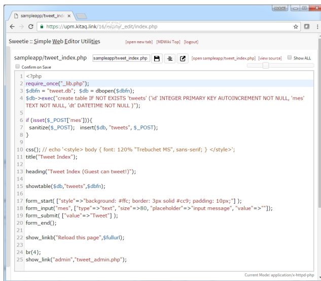
図 2 Tweet Index のソースコード
